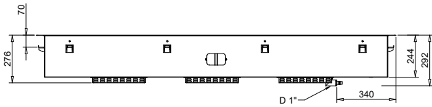
Zij aanzicht
