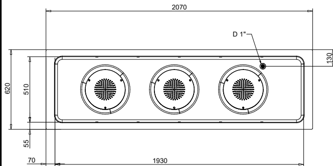
Boven aanzicht
